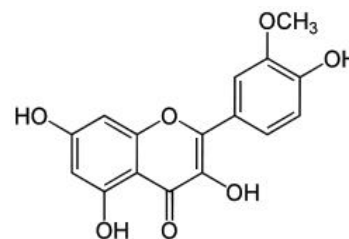
Рисунок 5 – УФ-спектр и структурная формула изорамнетина
